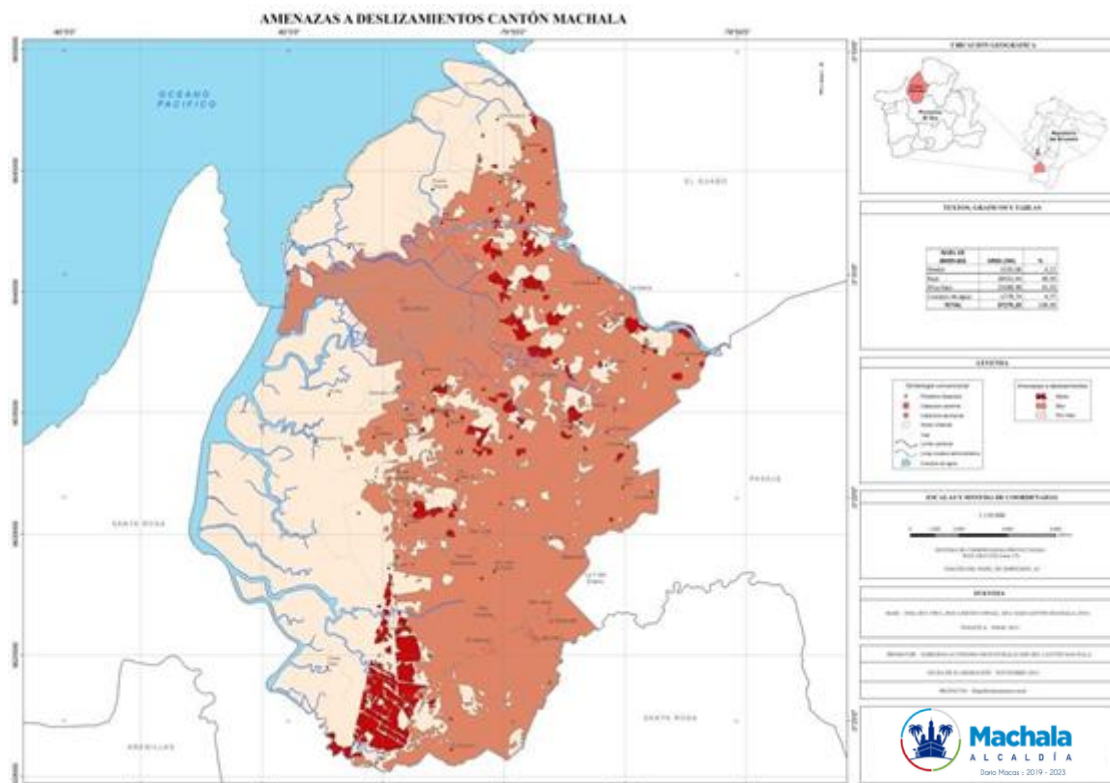
Mapa 18: Movimientos en masa – Susceptibilidad
