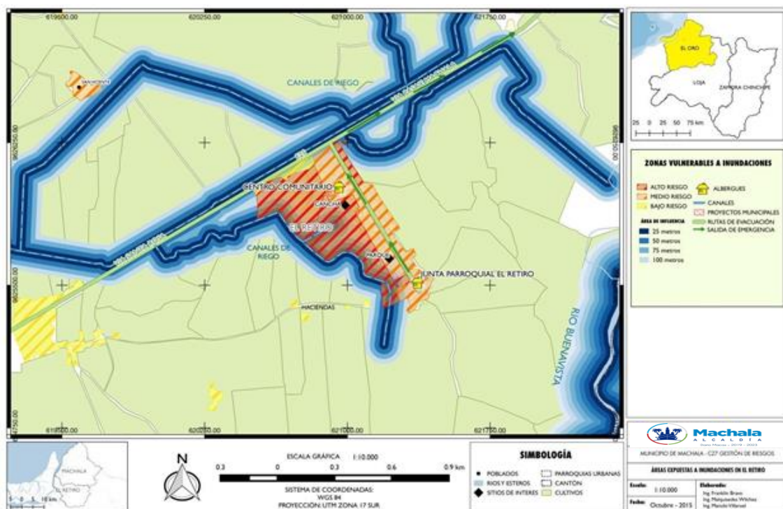
Esquema 2: Riesgo de inundaciones sector urbano El Retiro
