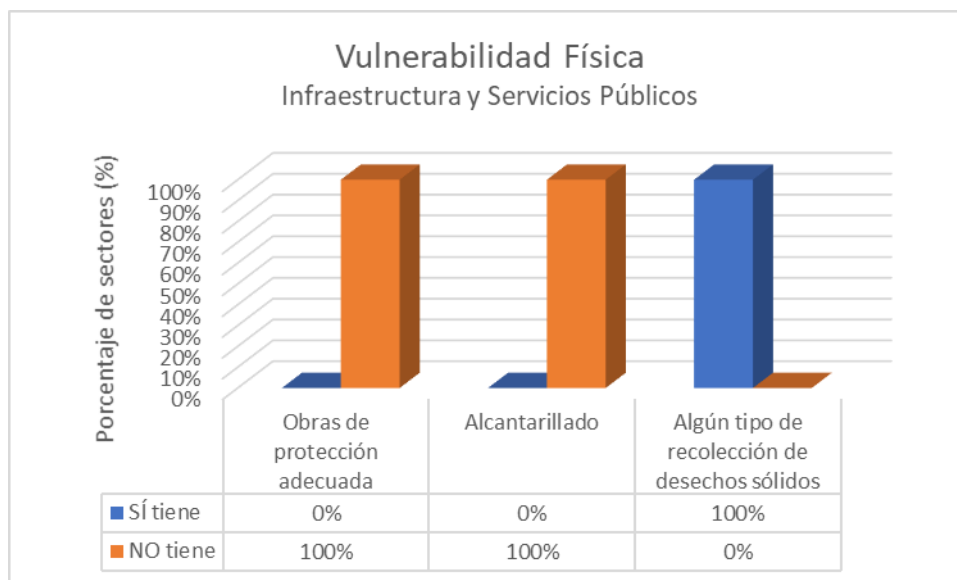
Ilustración 12: Vulnerabilidad física
