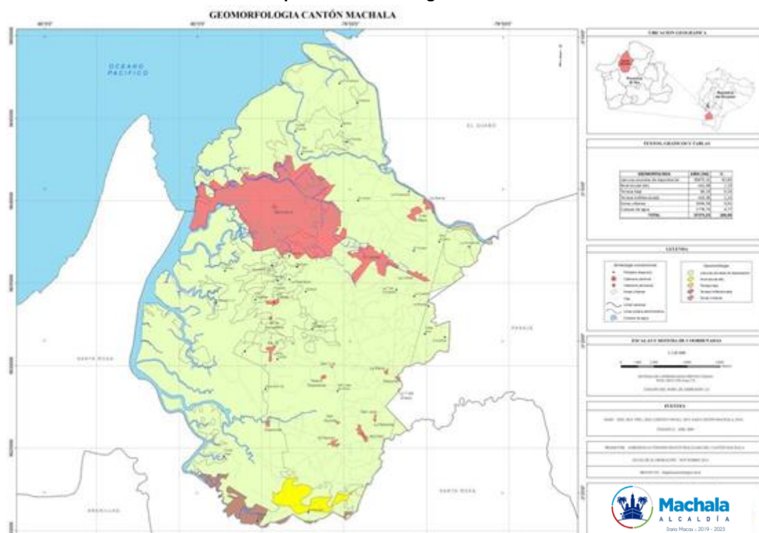
Mapa 17: Geomorfología Machala
