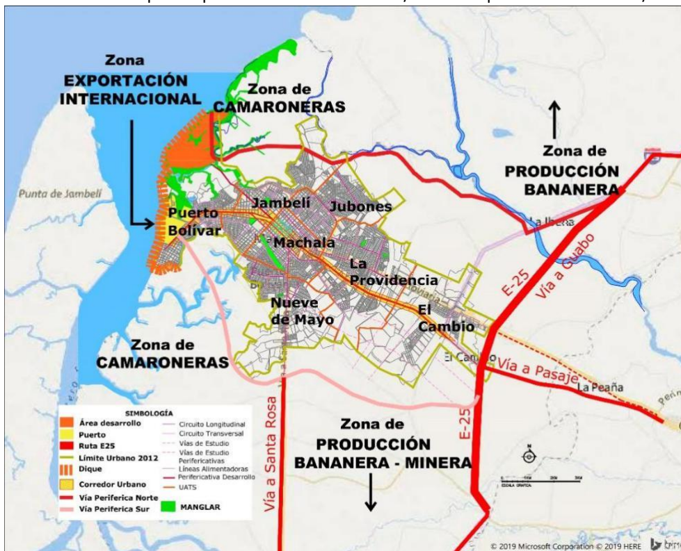
Esquema 14: Red Vial Propuesta para la ciudad de Machala / Zonas de producción actuales / Conexiones
