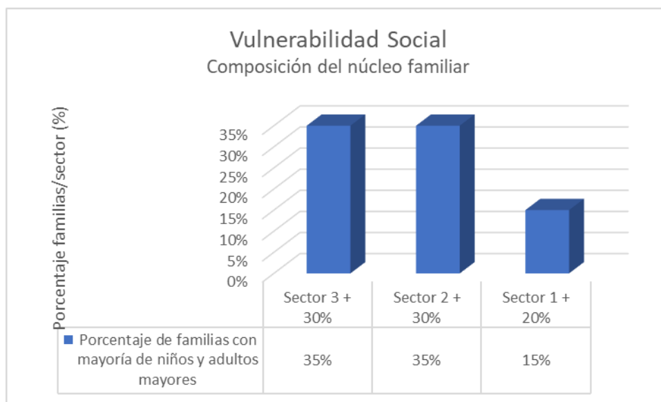
Ilustración 13: Vulnerabilidad Social
