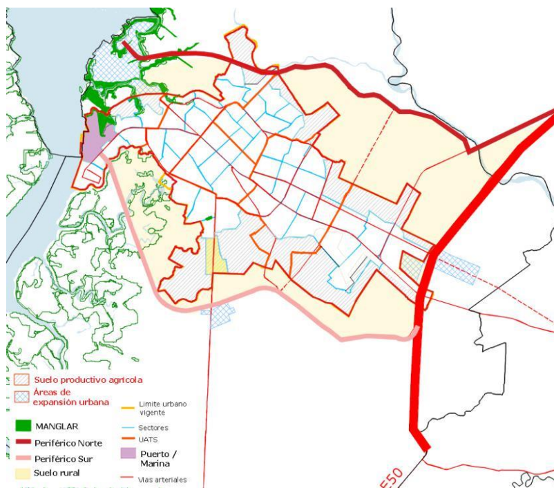
Esquema 19: Estructura territorial según sistemas viales
